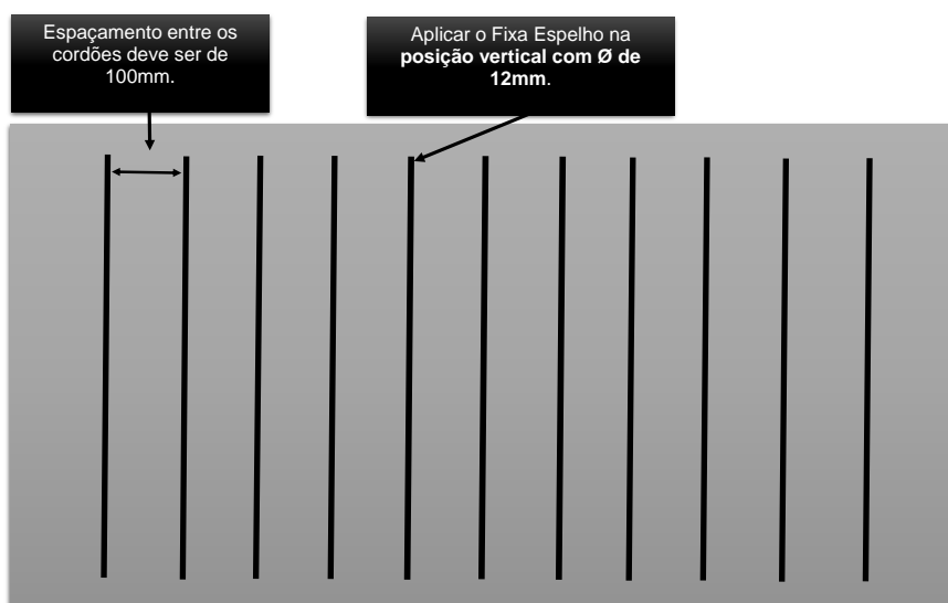
Figura 1 - Tamanho e espaçamento do cordão do produto (selante).
